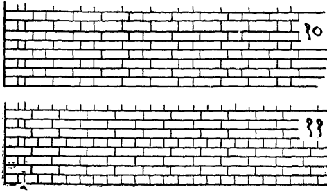
१०. Garden wall bond : गार्डन वॉल ११. Facing bond : फेसिंग
